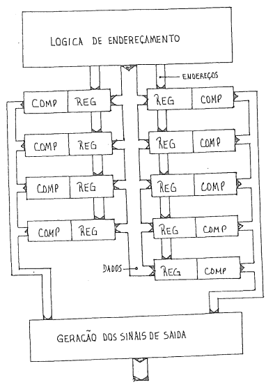
Figura 2: Arquitetura Interna.
