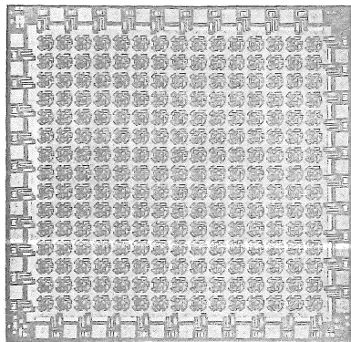
FIGURA 2.- UM "GATE-ARRAY" ANTES E DEPOIS DA PERSONALIZAÇÃO (ref. 6)
