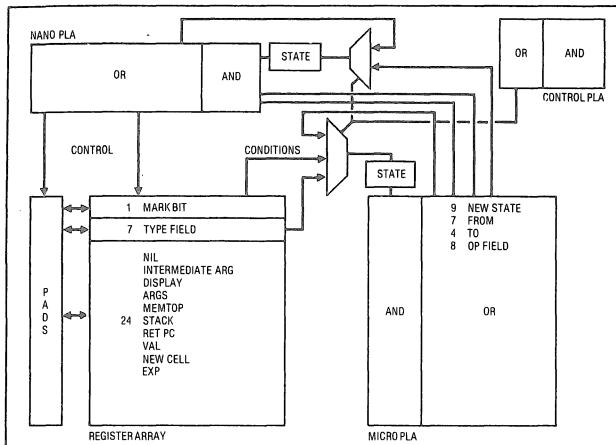
Figure 6: MIT Scheme-79 Machine Organisation
