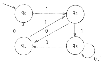
Fig. 1 - Autômato finito determinístico que detecta dois 0's ou dois 1's consecutivos.
