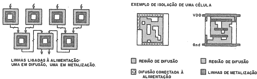
Figura 4: Restrições de isolação (regra 2)
